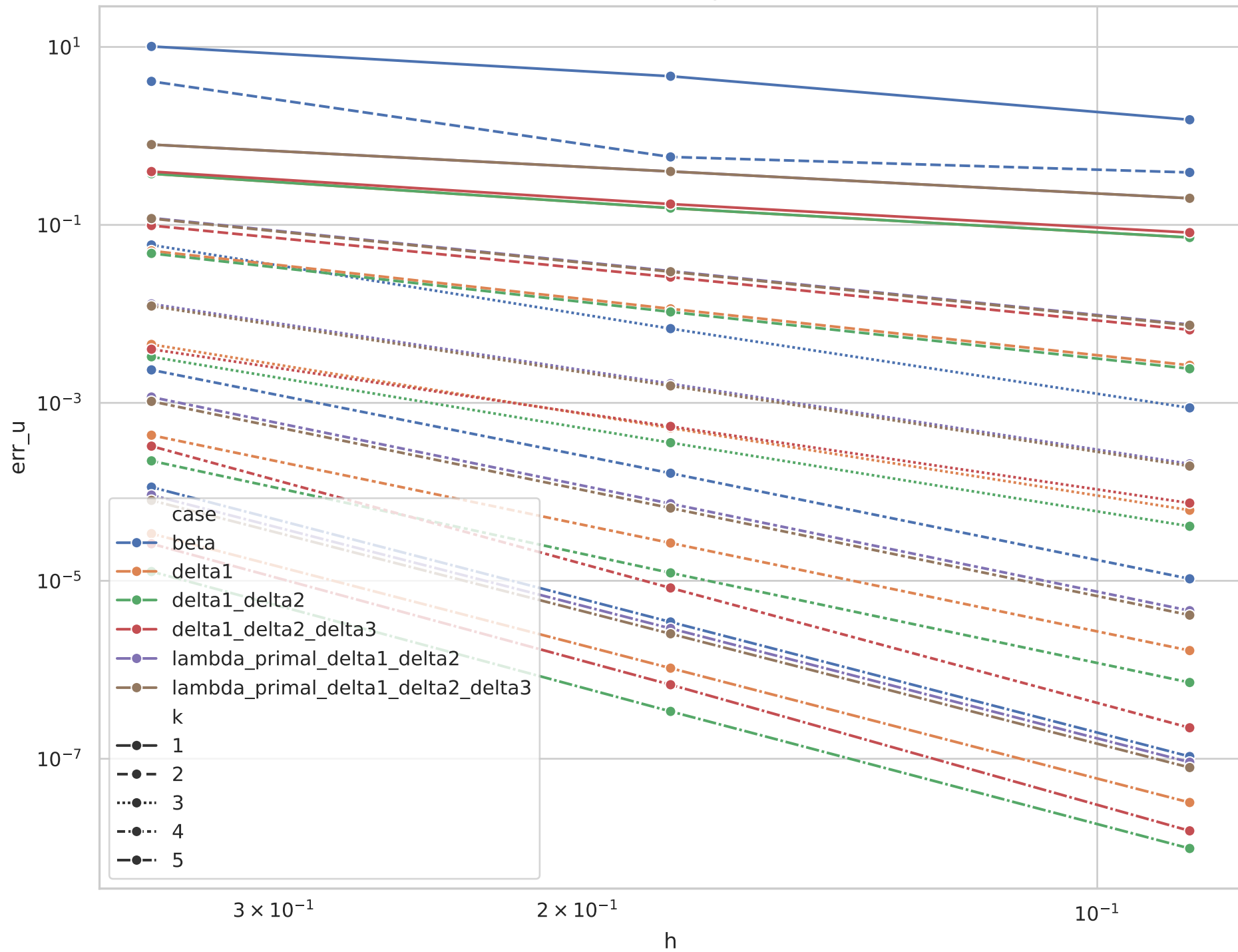
Lista 3 2D - convergência de u
